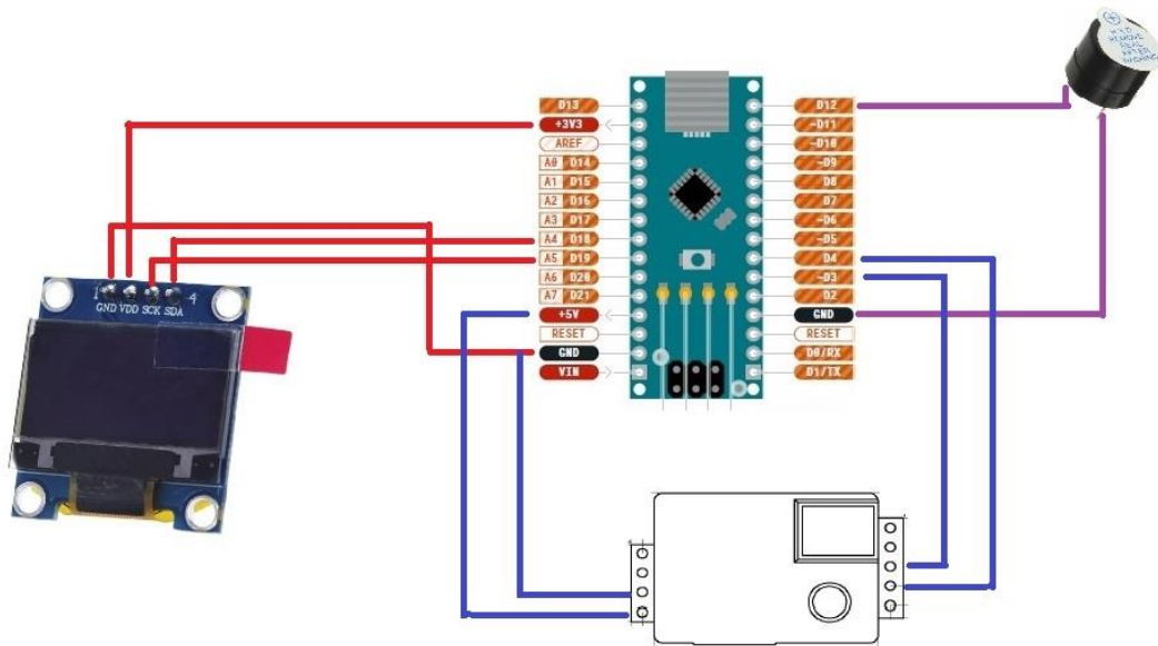
DIAGRAMA DEL CIRCUITO
