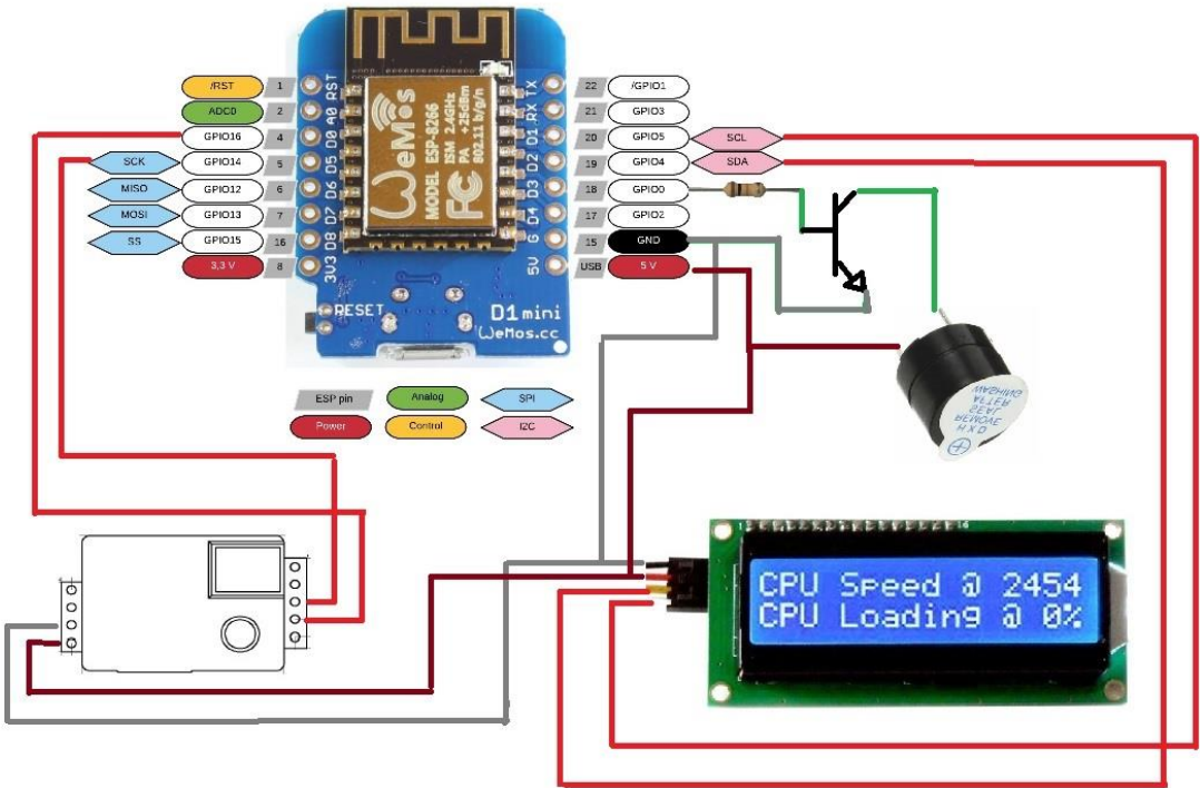
DIAGRAMA DEL CIRCUITO
