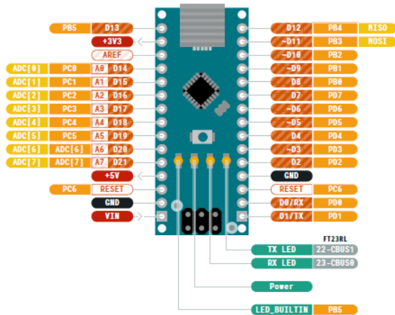
DIAGRAMA DEL ARDUINO NANO
